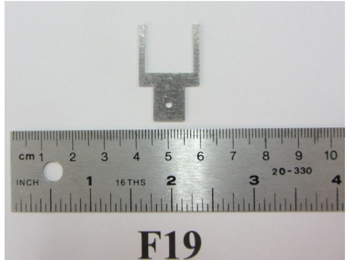
Fig. 10e: Type F19 fork.
